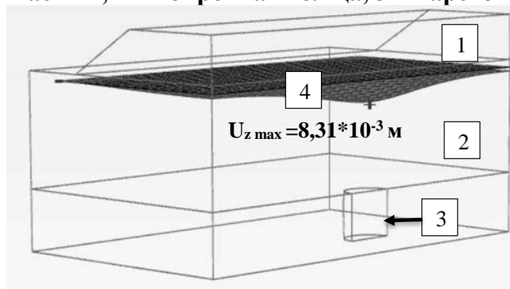
Рисунок 7 – Деформации геосинтетического материала при образовании карстовой полости, где 1 – дорожная насыпь, 2 – покровная толща, 3 – карстовая полость, 4 – эпюра вертикальных перемещений геоматериала
