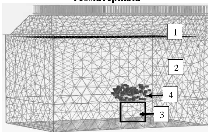
Рисунок 8 – Образование «свода обрушения» в грунтах покровной толщи при развитии карстовой полости в карстующихся грунтах, где 1 –
