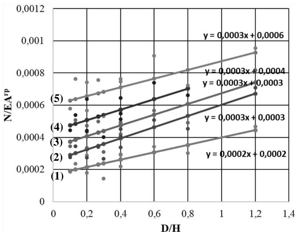
Рисунок 9 – График зависимости усилий в геоматериале ( N ) от жесткости геоматериала, взаимодействующего с грунтом ( EA_{гр} ), диаметра полости D и мощности покровной толщи ( H ) при высоте насыпи ( h ): 2 м – (1), 3 м – (2), 4 м – (3), 5 м – (4), 6 м – (5)
