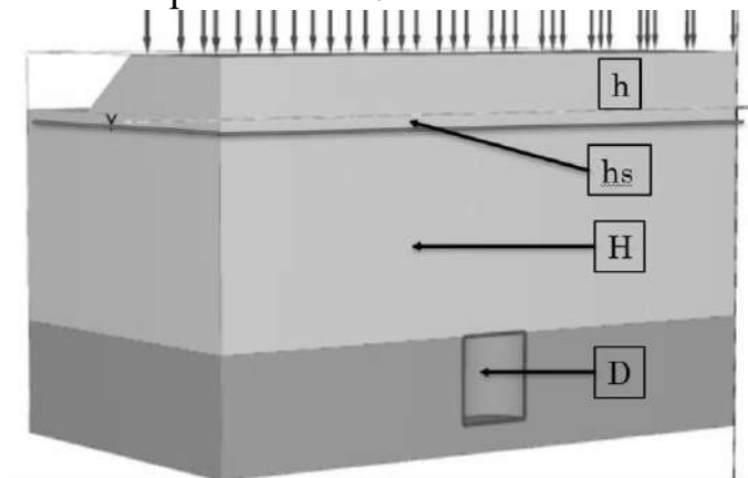
Рисунок 5 – Расчетная модель численных исследований
