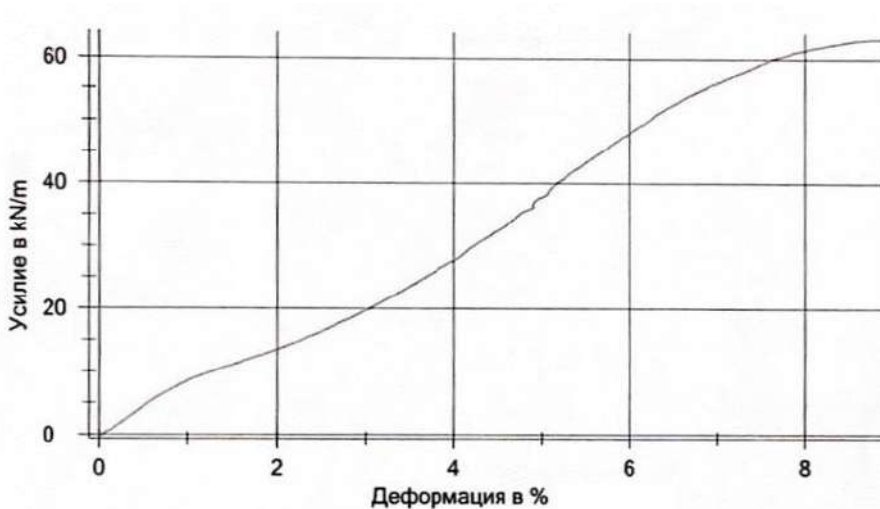
Рисунок 3 – Результаты испытания в разрывной машине. График зависимости растягивающих усилий от деформаций для геосинтетического материала Huesker Stabilenka 400 в поперечном направлении
