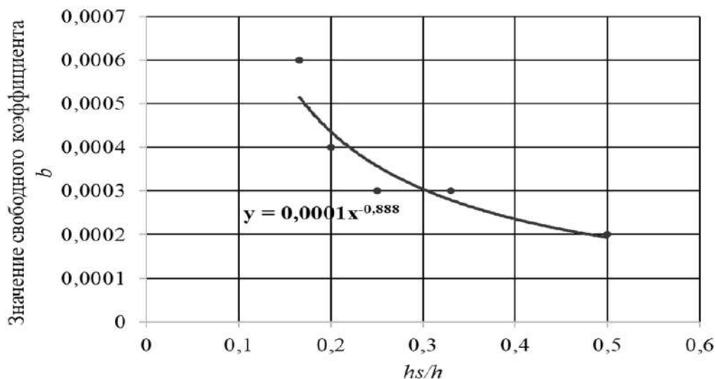
Рисунок 10 – График зависимости коэффициента b от h_s/h
