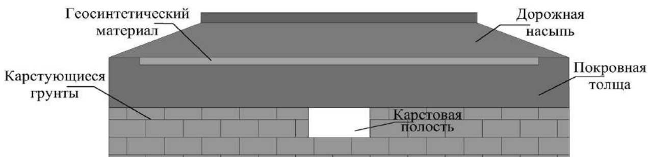
Рисунок 1 – Армированная дорожная насыпь над полостью в карстующихся грунтах
