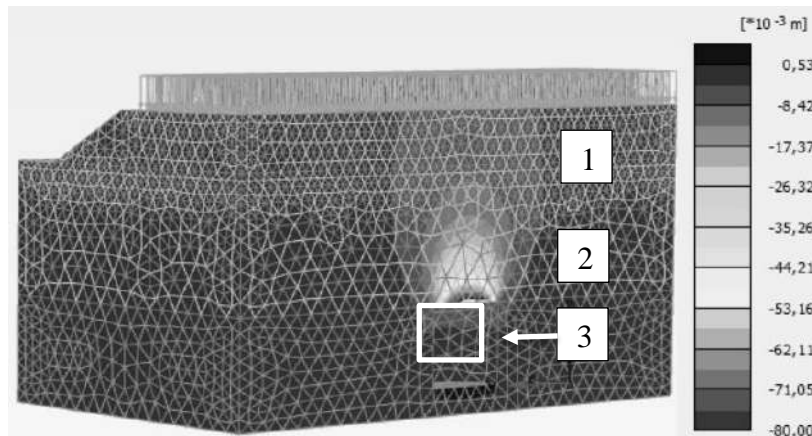
Рисунок 6 – Вертикальные перемещения грунта покровной толщи и насыпи автомобильной дороги при образовании карстовой полости, где 1 – дорожная насыпь, 2 – покровная толща, 3 – карстовая полость
