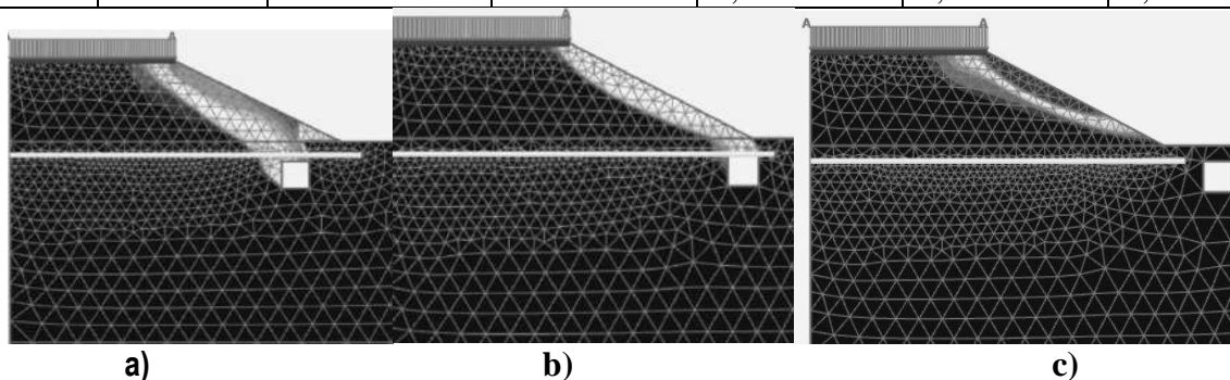
Рисунок 12 – Поверхности сдвига при образовании карстового провала: а) провал под откосом; б) провал в основании откоса; с) провал за основанием откоса
