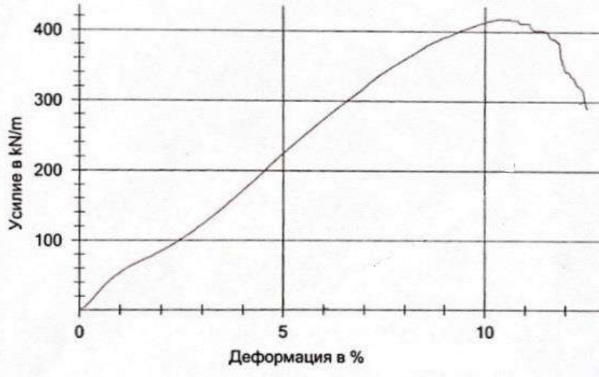
Рисунок 2 – Результаты испытания в разрывной машине. График зависимости растягивающих усилий от деформаций для геосинтетического материала Huesker Stabilenka 400 в продольном направлении
