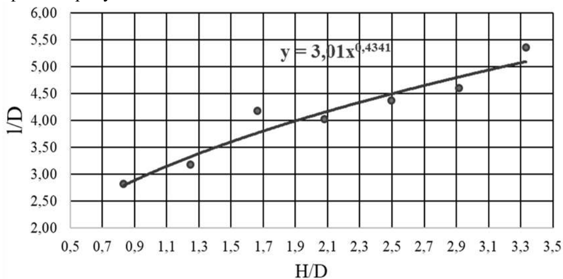
Рисунок 11 – Зависимость размера мульды проседания от диаметра полости и толщины покровной толщи
