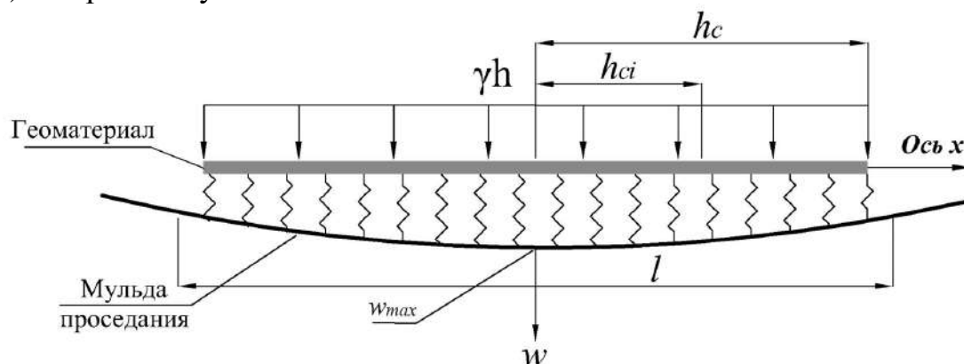
Рисунок 13 – Расчетная схема
